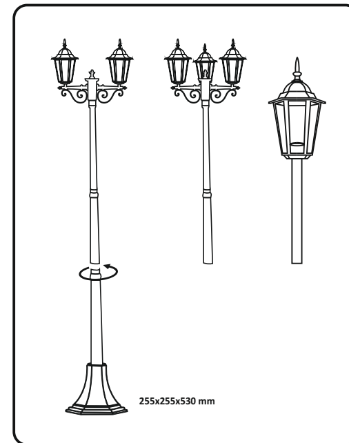
max 60W E27; IP43; 220-240V ~50/60Hz
